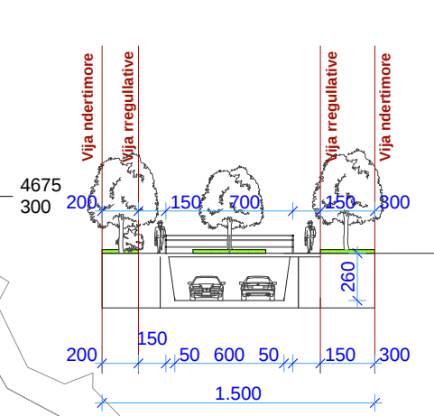
Profili 4-4
