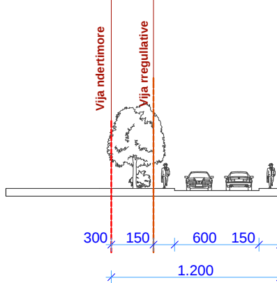
Profili 5-5
