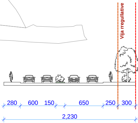
Profili 7-7
