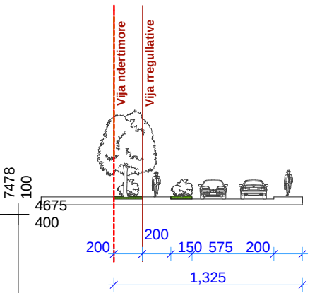
Profili 2-2
