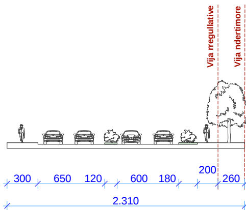
Profili 3-3
