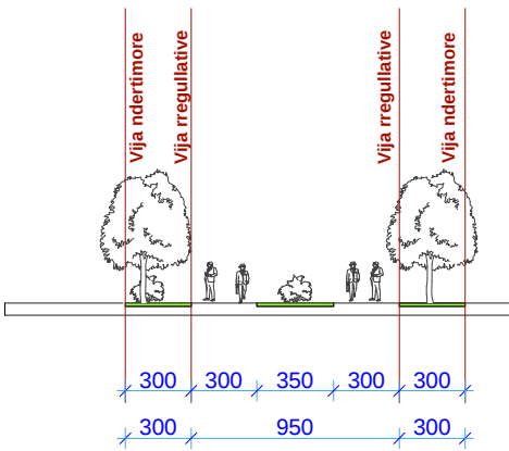
Profili 1-1
