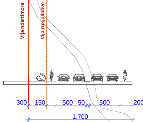
Profili 6-6
